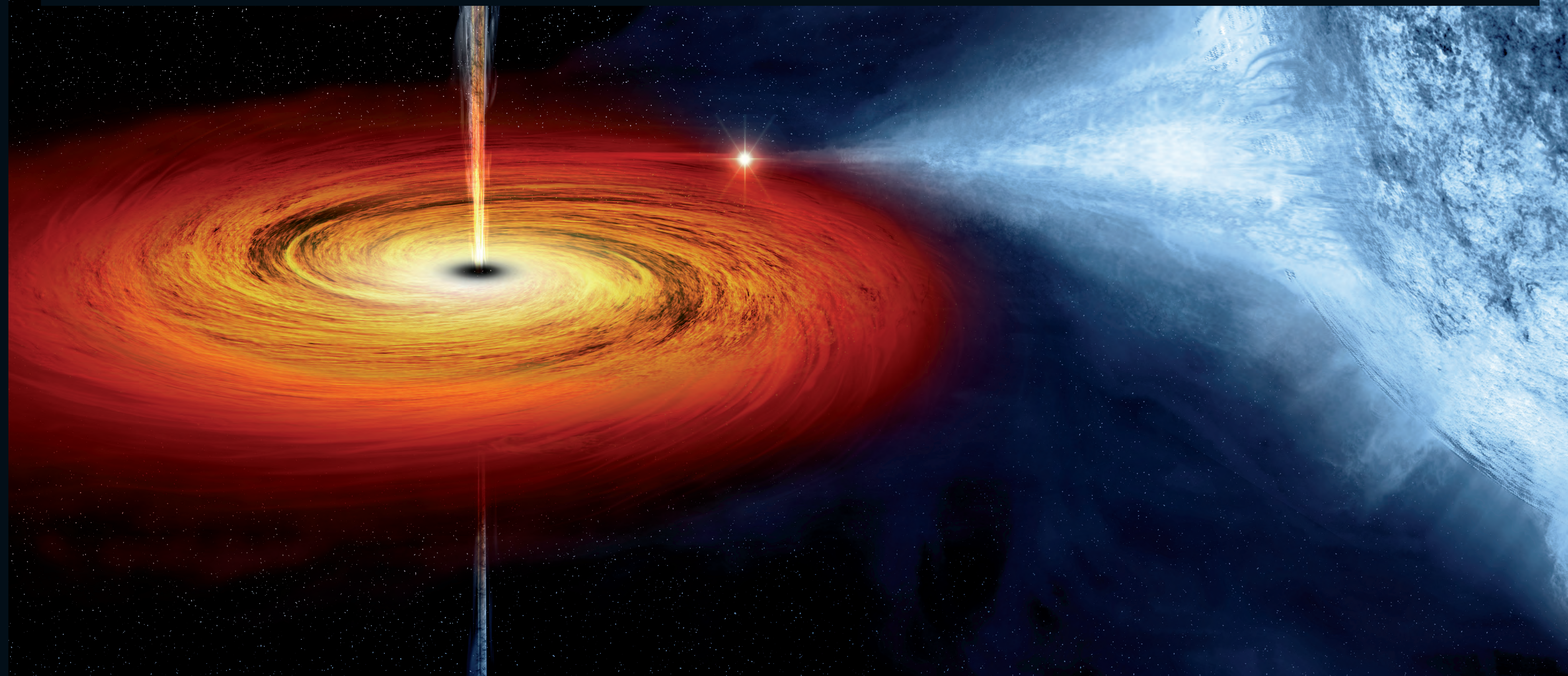
Il·lustració artística del sistema Cygnus X-1. El forat negre atrau cap a ell matèria provinent d'una estrella companya blava. La matèria o bé forma un disc abans de caure al forat negre o bé n'és expulsada en forma de potents raigs de matèria. (NASA/CXC/M.Weiss)
